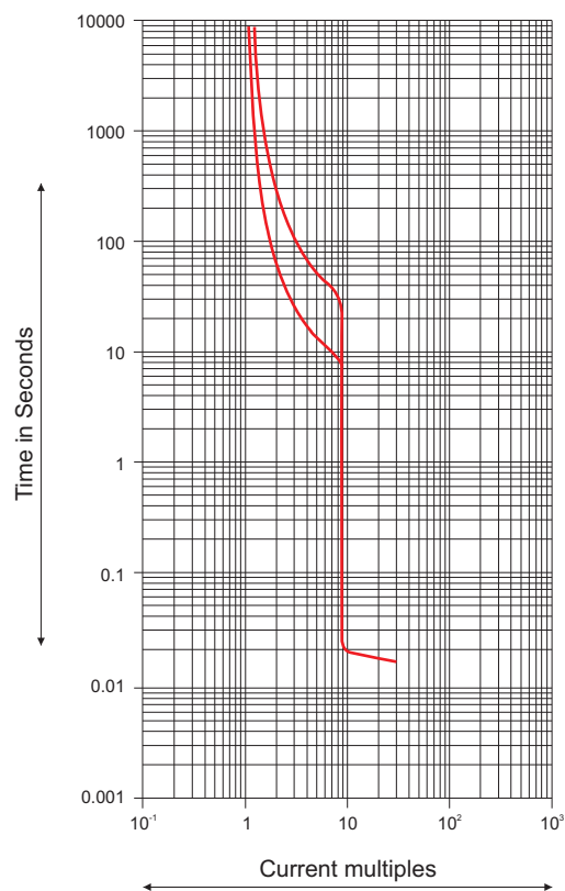
DU250
