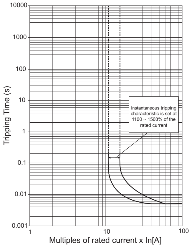
Type MOG - H2M (32A - 63A)
